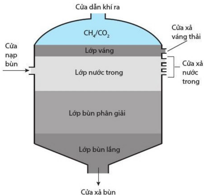
Hình 12.6. Xử lý nước thải kỵ khí
