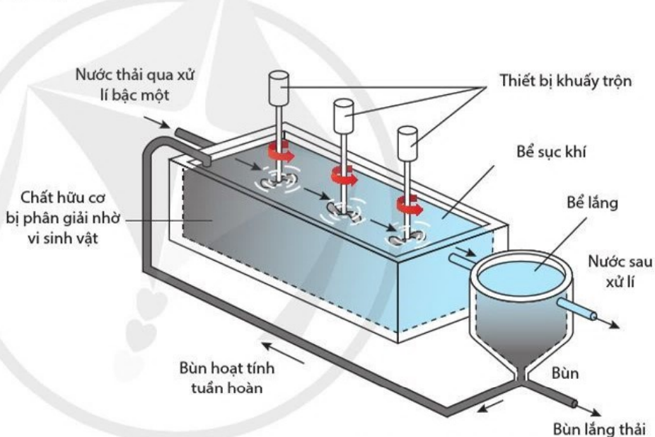
Hình 12.7. Hệ thống bùn hoạt tính hiếu khí
