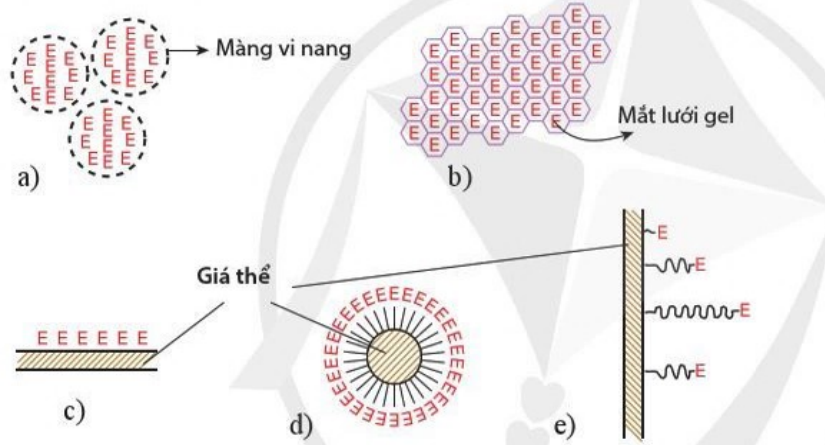
Hình 10.2. Các kỹ thuật cố định enzyme (chú thích: E – enzyme)
