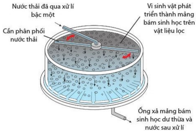
Hình 12.8. Hệ thống lọc nhỏ giọt
