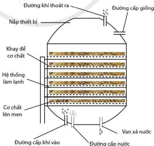
Hình 8.5. Hệ thống nuôi cấy bề mặt rắn
