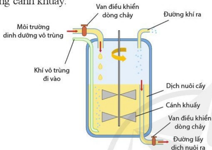
Hình 8.6. Hệ thống nuôi cấy chìm liên tục
