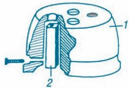
Hình 51.6. Ổ điện 1. Vỏ ; 2. Cực tiếp điện.
