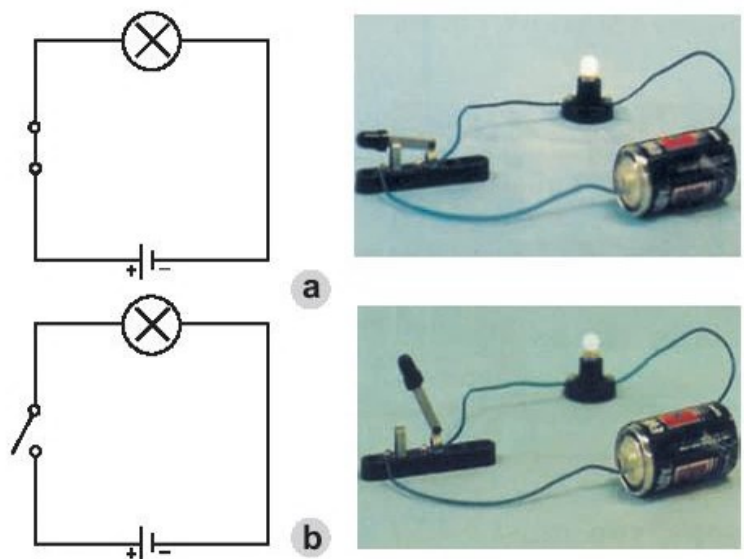
Hình 51.1. Mạch điện chiếu sáng
