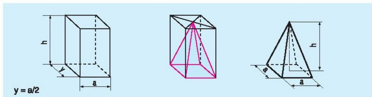
Hình 5.5. Cách vẽ hình chóp
