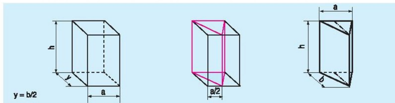
Hình 5.4. Cách vẽ hình lăng trụ
