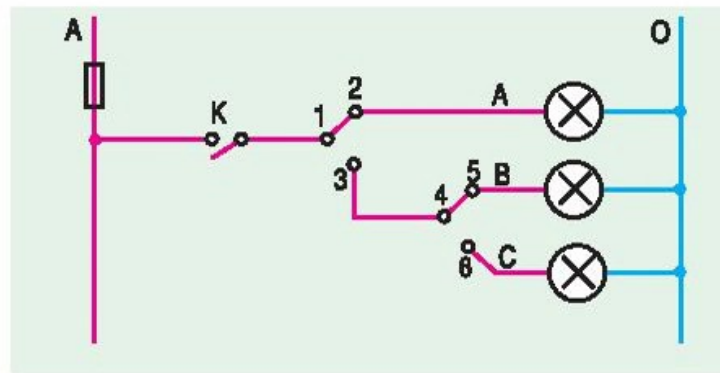
Hình 2. Mạch điện chiếu sáng xoay chuỗi
