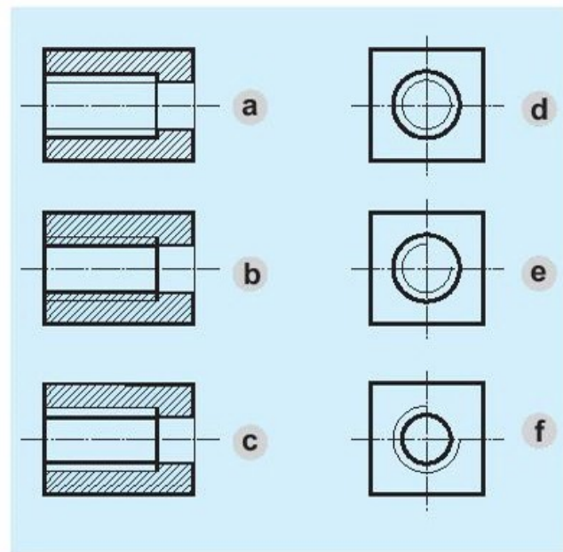
Hình 11.8. Ren lỗ
