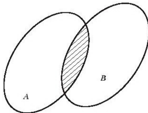
A \cap B Hình 5
