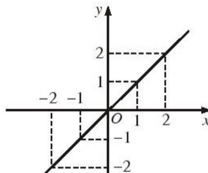
Đồ thị hàm số y = x
