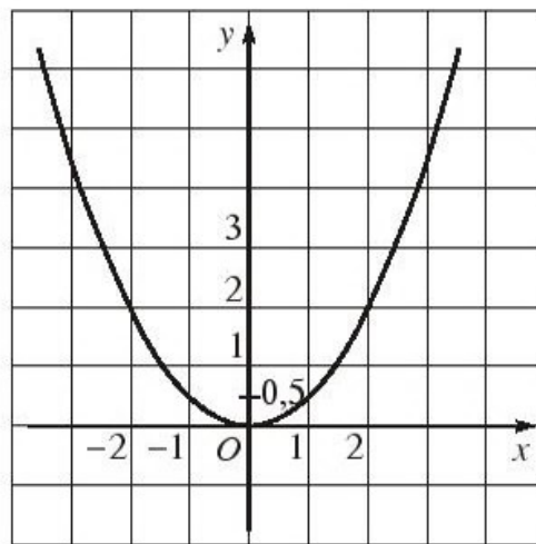
Đồ thị hàm số g(x) = \frac{1}{2}x^2
