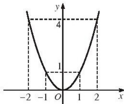
Đồ thị hàm số y = x^2
