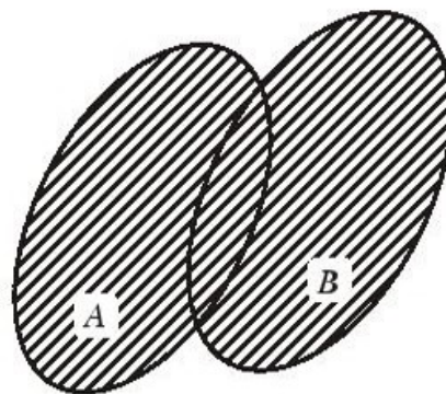
A \cup B Hình 6
