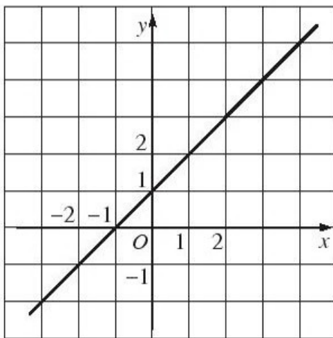
Đồ thị hàm số f(x) = x + 1
