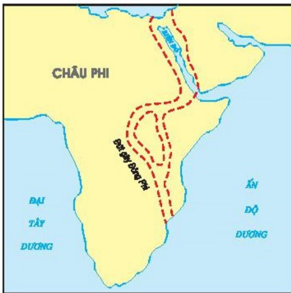
Hình 8.4 – Đứt gãy Đông Phi và Biển Đỏ
