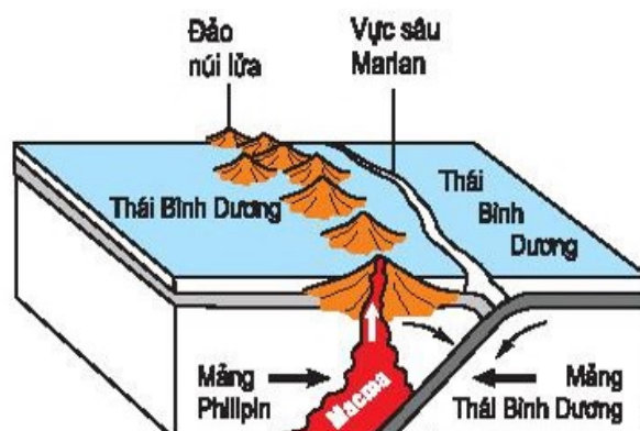
Hình 7.5 – Hai mảng kiến tạo xô vào nhau.
