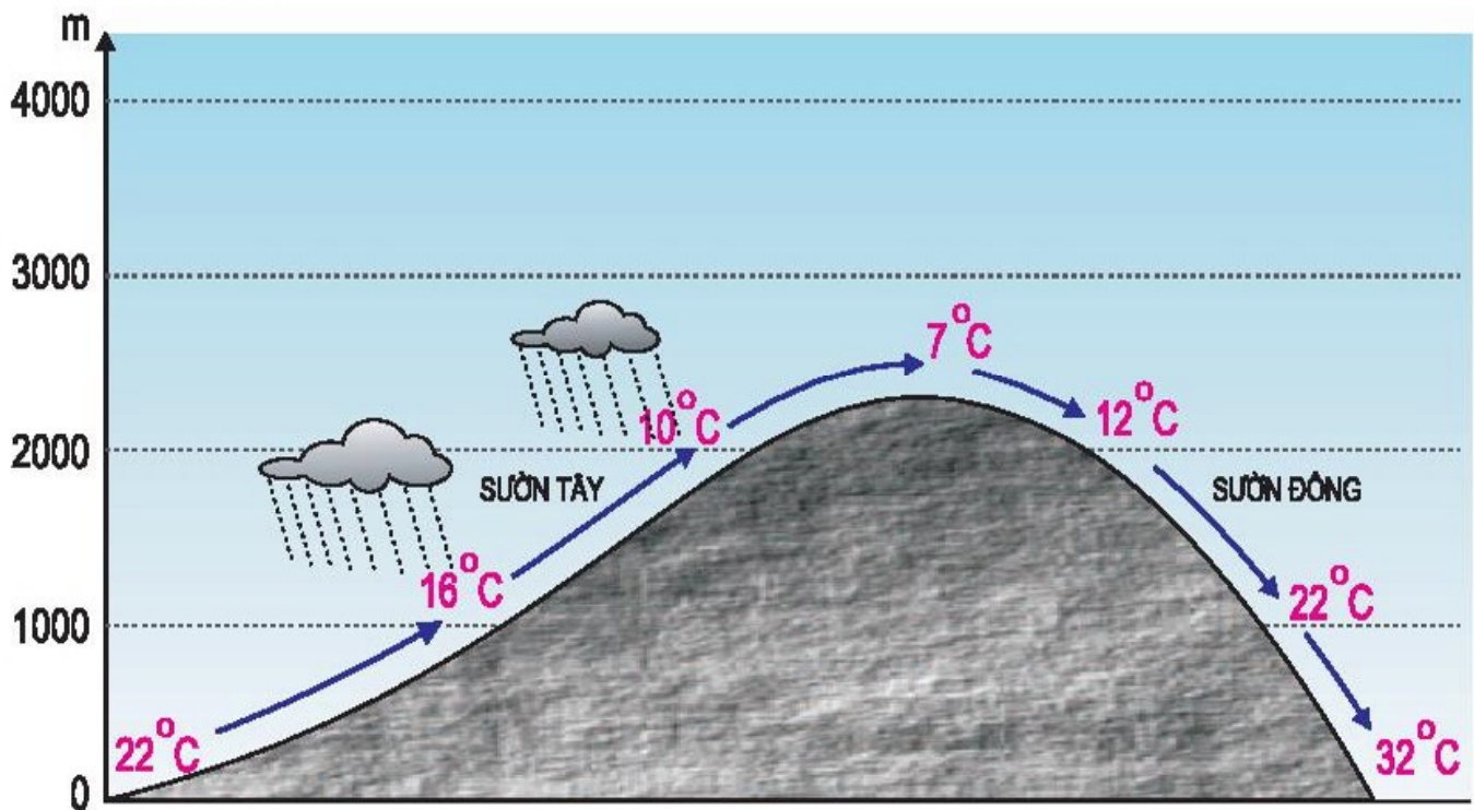
Hình 12.5 – Quá trình hình thành gió fơn
