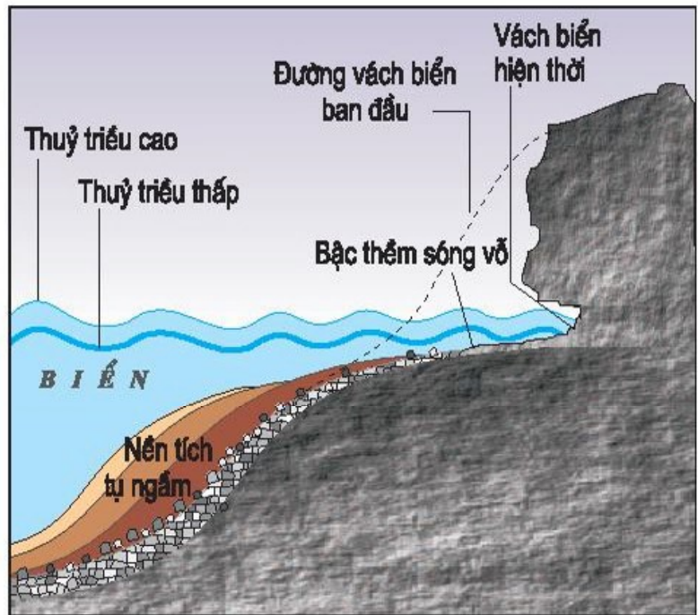
Hình 9.6 – Vách biển và bậc thềm sóng vỗ
