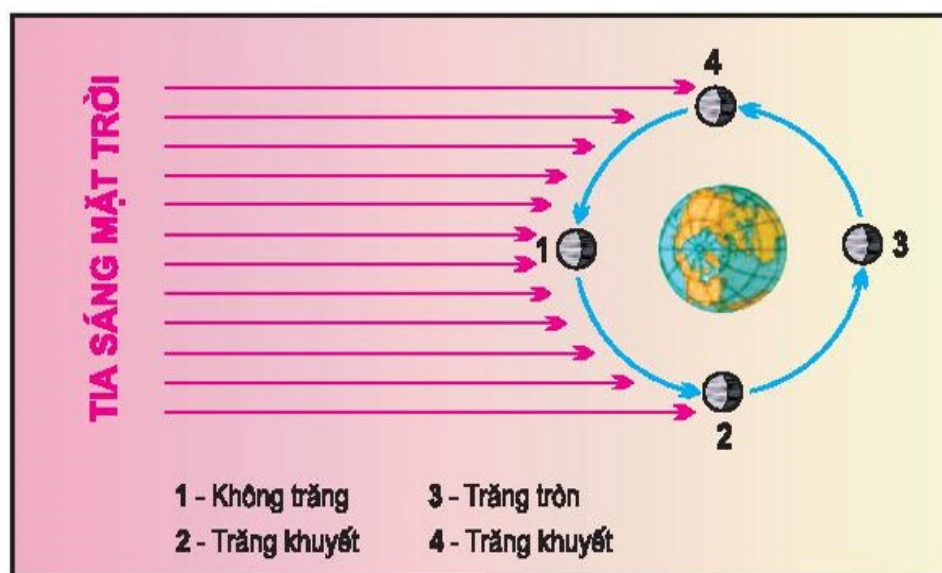
Hình 16.1 - Chu kì tuần trăng
