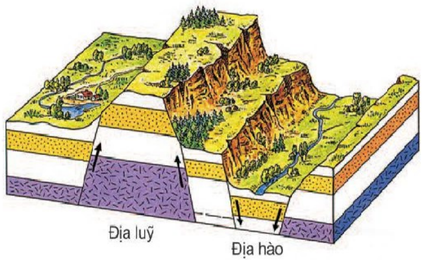
Hình 8.3 – Địa lũy và địa hào
