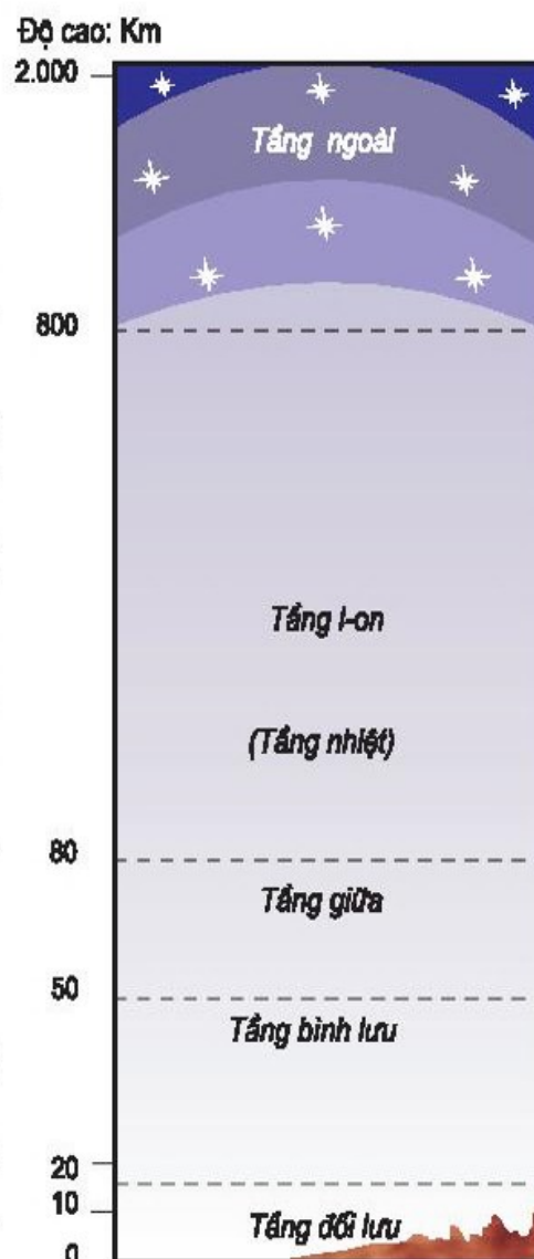
Hình 11.1 – Các tầng khí quyển
