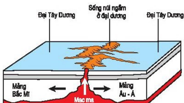
Hình 7.4 – Hai mảng kiến tạo tách rời nhau.
