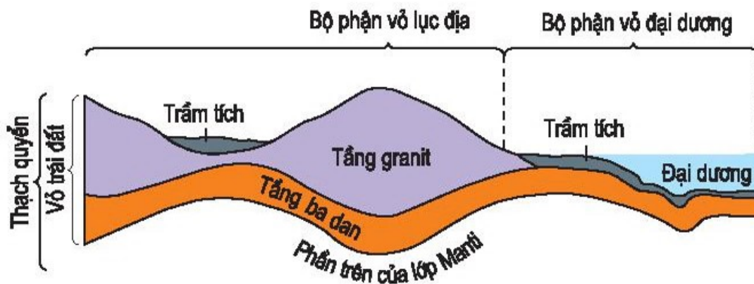
Hình 7.2 – Lớp vỏ Trái Đất. Thạch quyển
