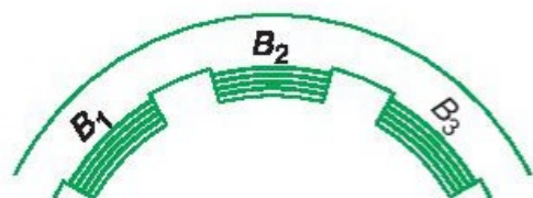
Hình 17.2 Các cuộn dây của phần ứng.
