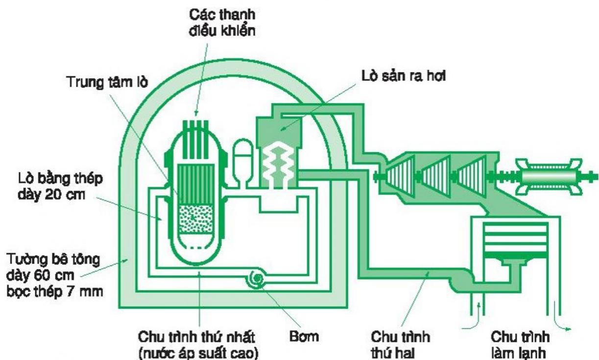
Hình 38.2. Sơ đồ lò phản ứng PWR.
