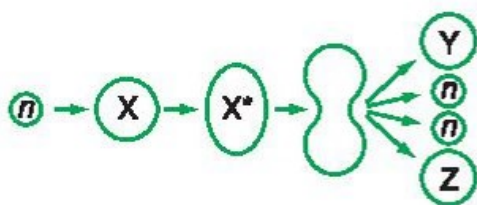
Hình 38.1 Sơ đồ phản ứng phân hạch
