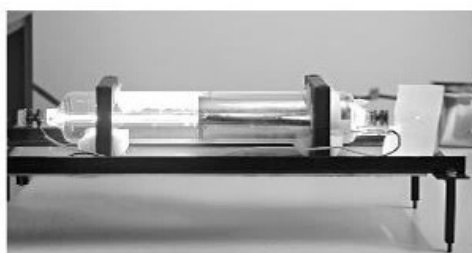
Hình 34.5 Laze khí
