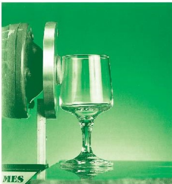
Cốc vỡ do hiện tượng cộng hưởng.
