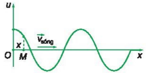
Hình 7.5 Sóng hình sin tại thời điểm t
